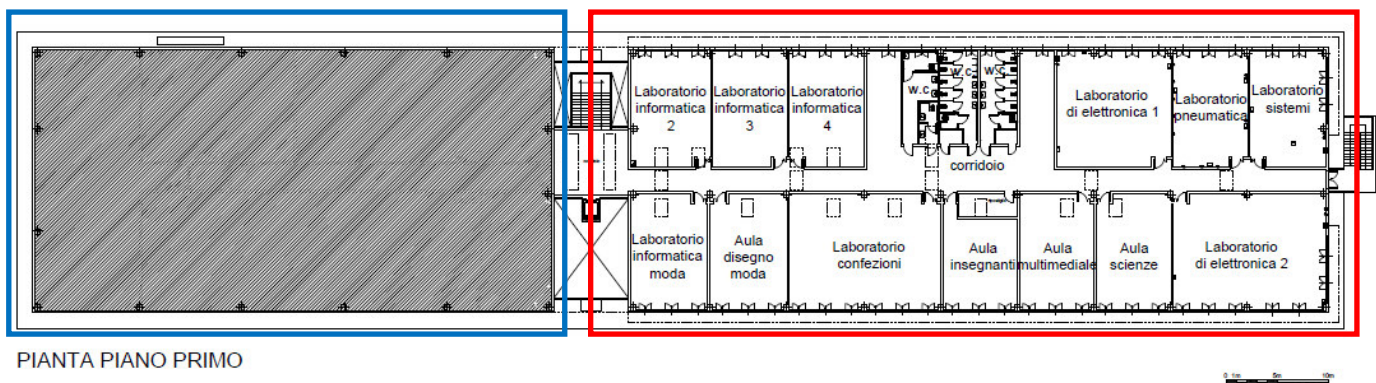
Planimetria di piano primo del complesso scolastico IPSIA "Ercole I d'Este"
